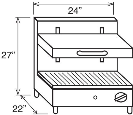
SEM-60 / SEM-80
